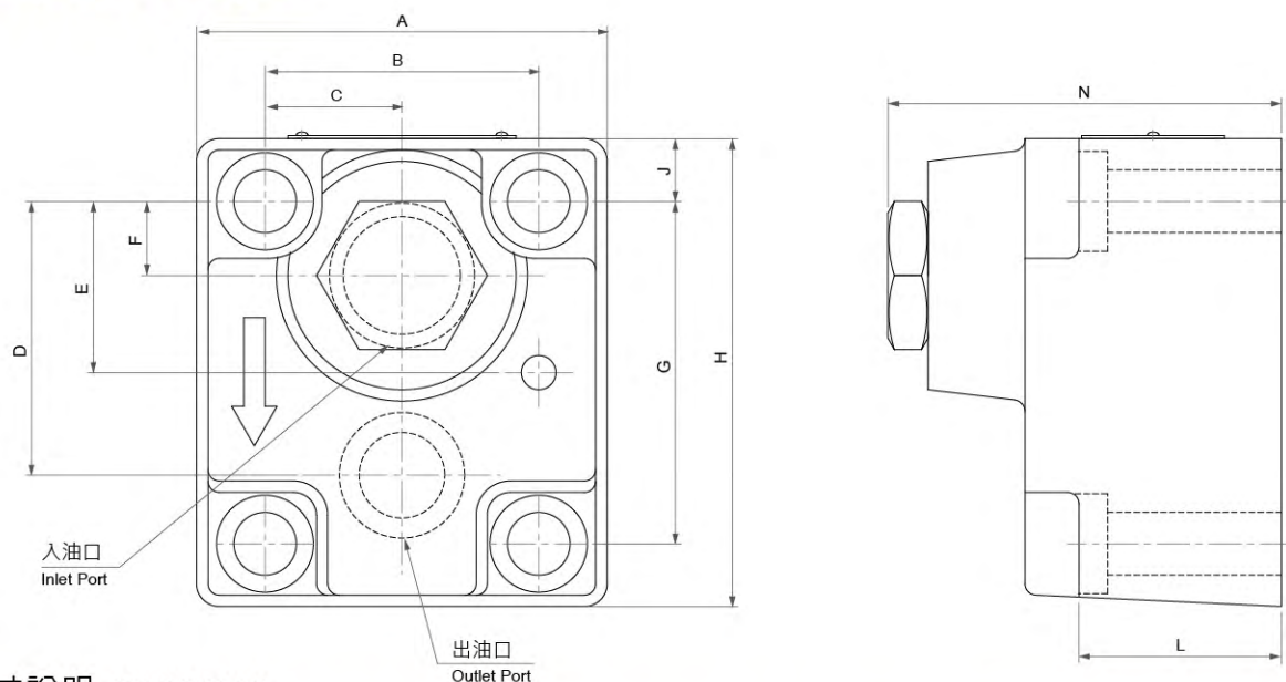
■ 尺寸說明 DIMENSION
